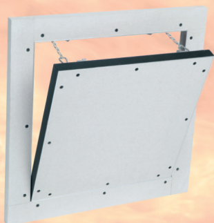
F5 EI30 per cavedio
