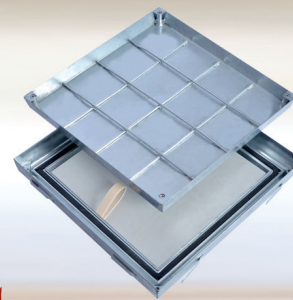
PRO+BS antincendio EI120
