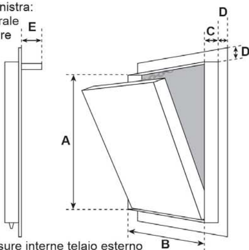
Variante 1: per il montaggio piastrelle sopra il telaio
